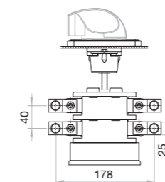
UL Terminal Lug
